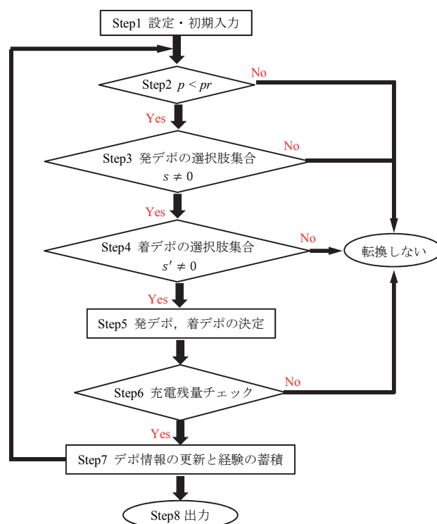
図-10 シミュレーションフロー
